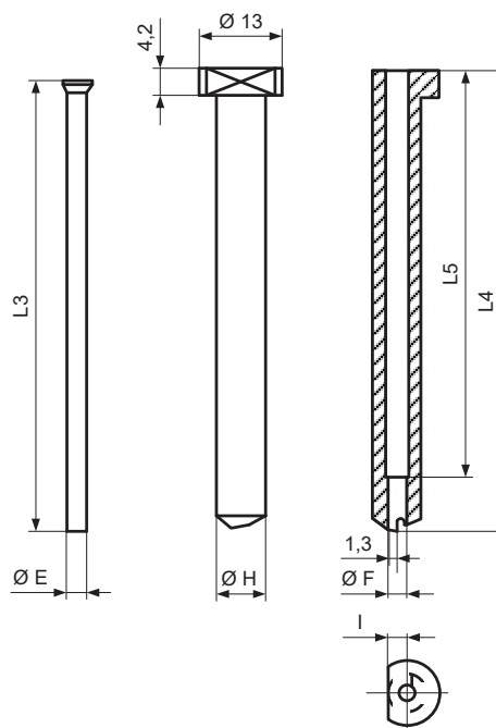
Stempel Punch
